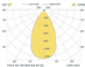
PACO-G2 60D
