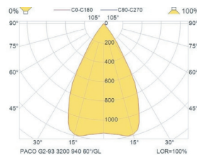
PACO-G2-93-3200-940-60-GL
