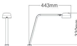
MOTUS-TABLE
